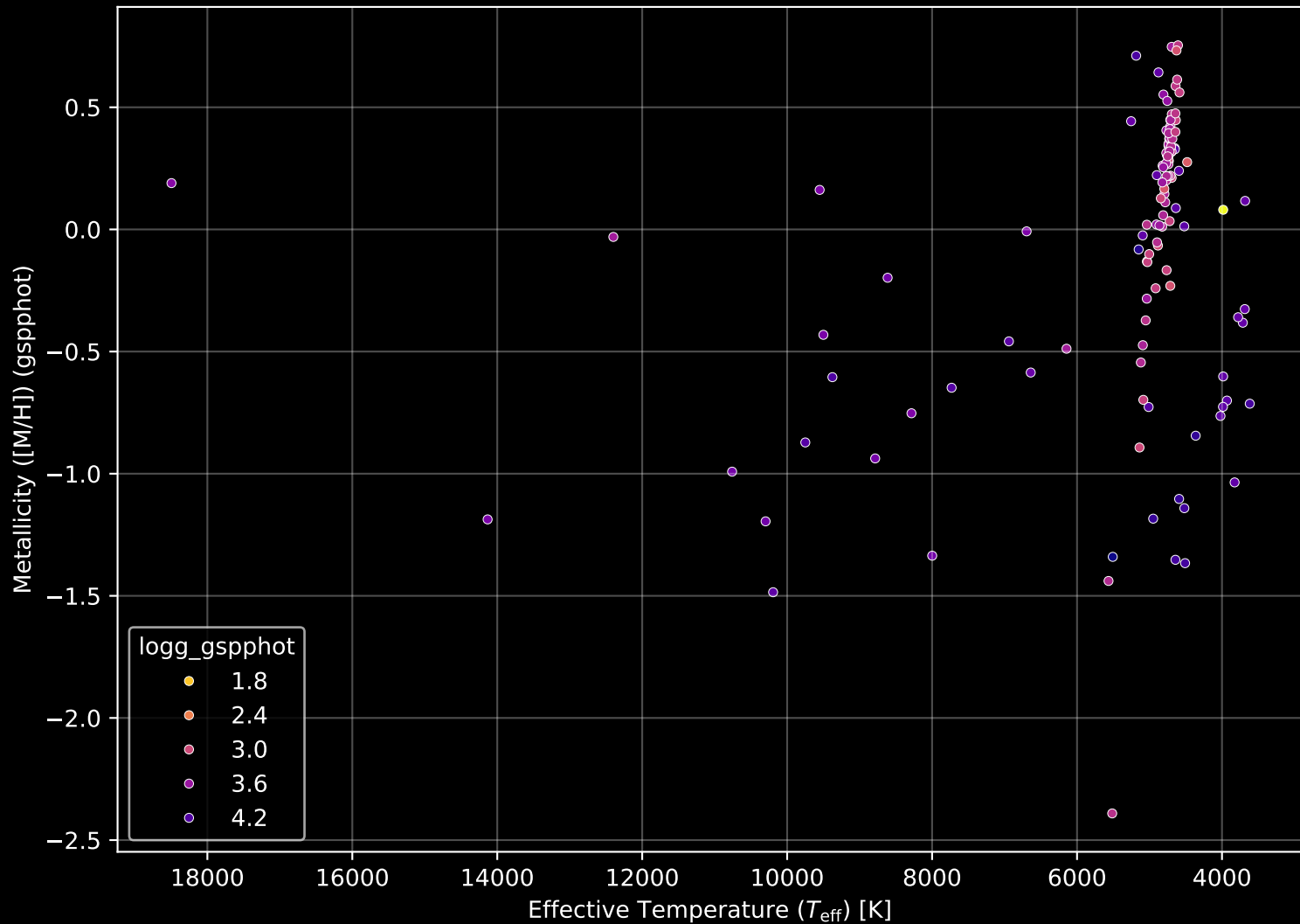
APOGEE DR17 Field: [033+00] Stellar Population Parameters (n= 123)
